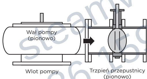
Rysunek 05: Pompa odśrodkowa (z wałem pompy w położeniu pionowym)
