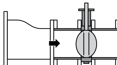
Haste da Válvula (Vertical)
