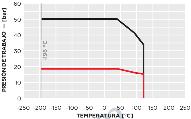
RELACIÓN (bar/°C) — ASME Clase 150 — Serie 40/41 — ASME Clase 300 — Serie 42/43
