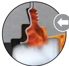
Pressão da linha aplicada na direção de fluxo não preferencial . (Durante ou após o evento de incêndio.)
