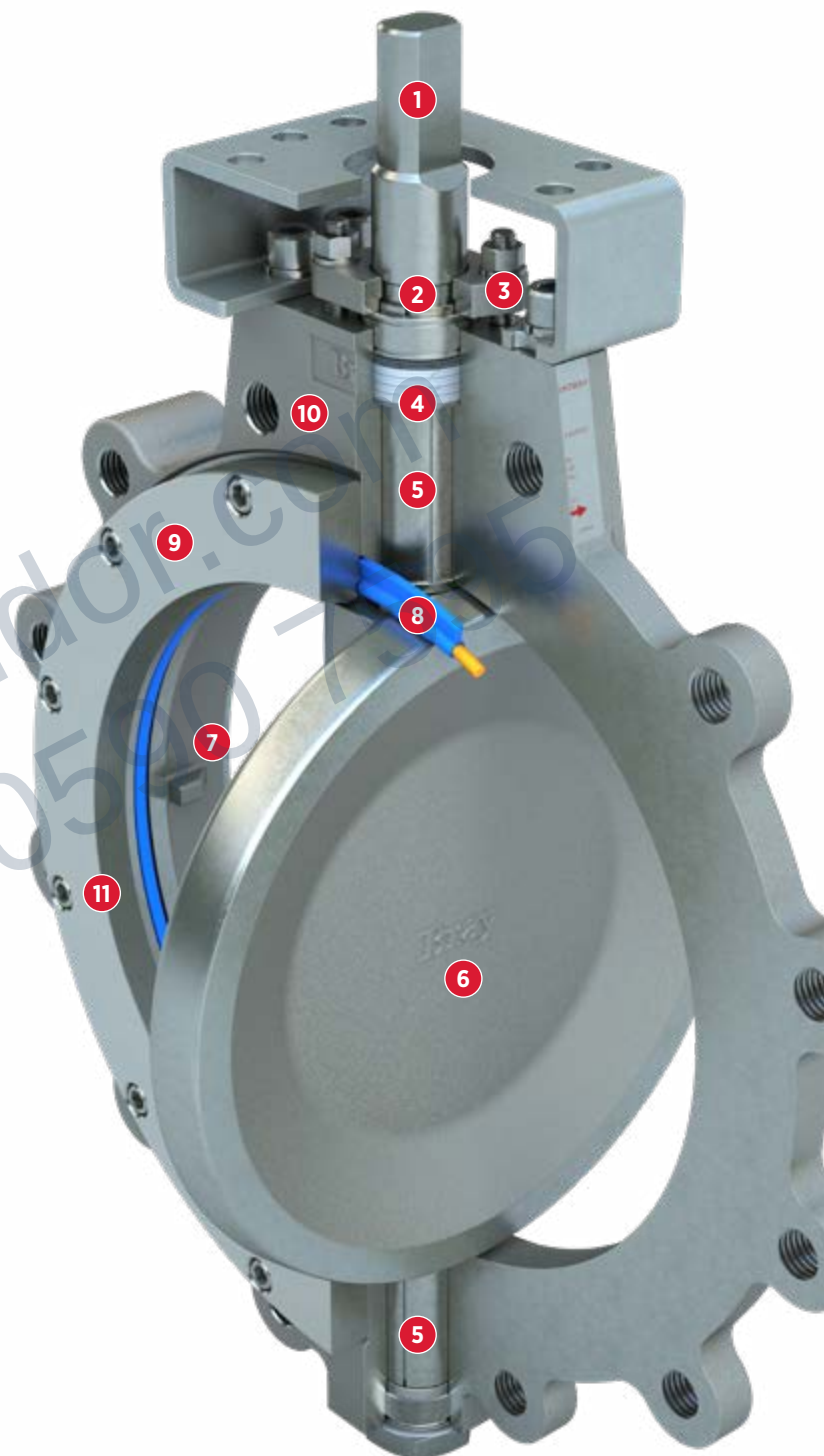
Estilo Lug Série 41
