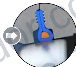
阀板处于关闭位置。 从首选流向施加的管线压力。
