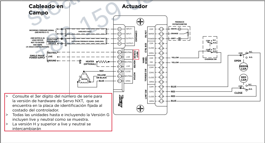
Figura 5 - Diagrama de cableado en campo de muestra para el actuador de la Serie 70 con Servo NXT.
