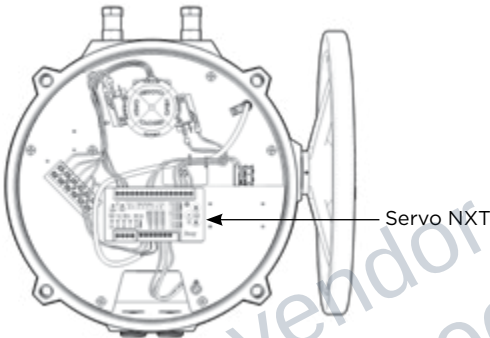
Figura 4 - S70 con Servo NXT
