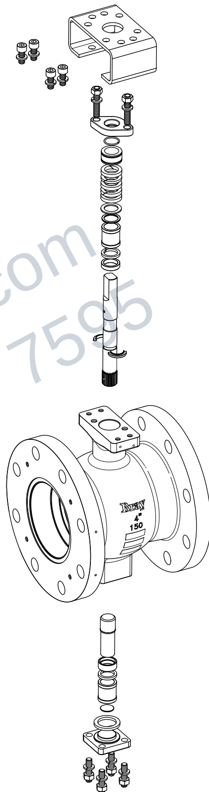
Obrázek 4: Demontáž ventilu.
