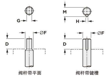
阀杆带平面
