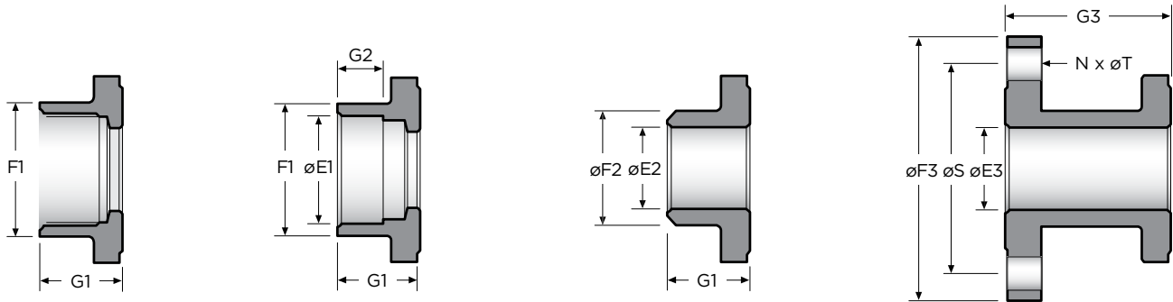
螺纹连接端盖 7100/8100
