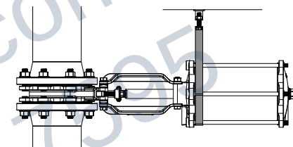
Figura 9: Soporte de instalación para una Válvula instalada con orientación Horizontal (Vástago en horizontal y Orificio en vertical)
