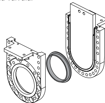
Figura 22: Afloje los sujetadores y separe las mitades del cuerpo de la válvula.
