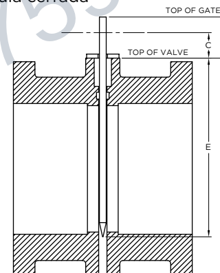
Figura 14: Ajuste de carrera, válvula cerrada
