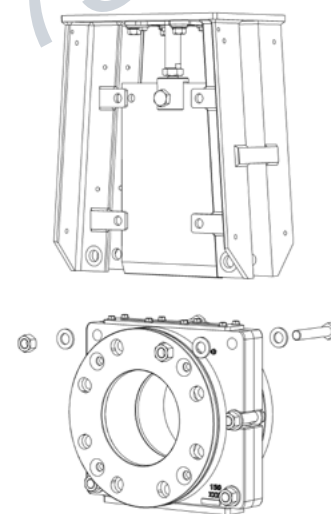
Figura 8: Desmontaje de la Compuerta
