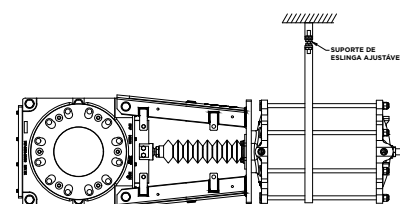
Figura 4: Válvula com Atuador
