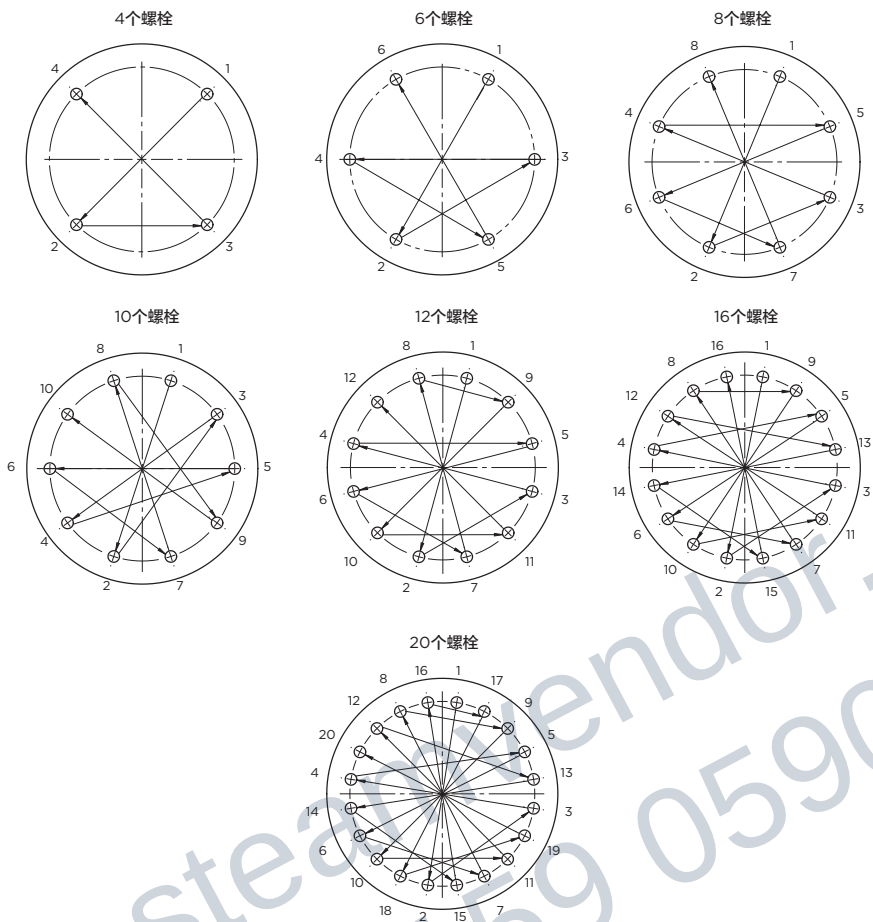
图4 - 阀体螺栓连接指南
