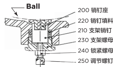
图1 - 球托结构
