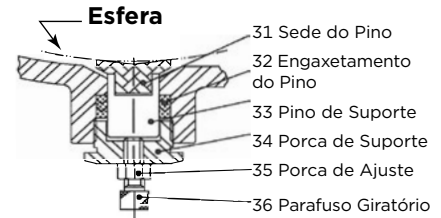
Suporte de Esfera
