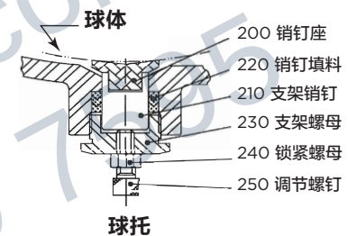
图1 - 球托结构
