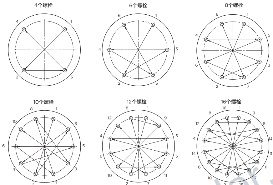
图4 - 阀体螺栓连接指南
