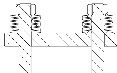
Figura 3 - Orientación de la Pila de Resortes Belleville del Bonete de la M1
