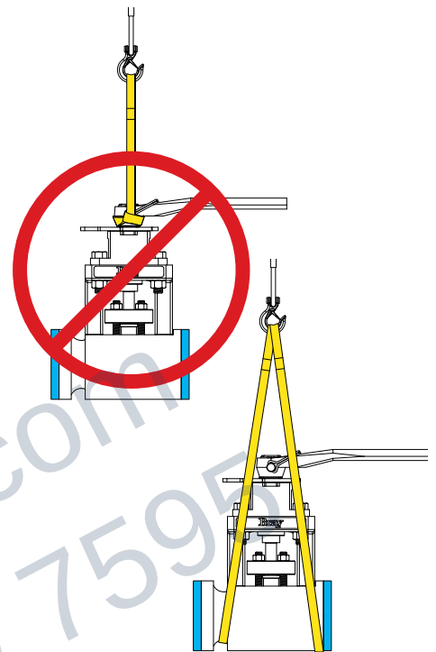
Figura 1: Válvula de elevación correcta con manija
