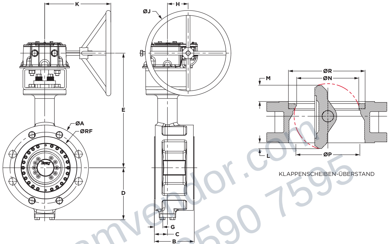
ABMESSUNGEN (mm)
