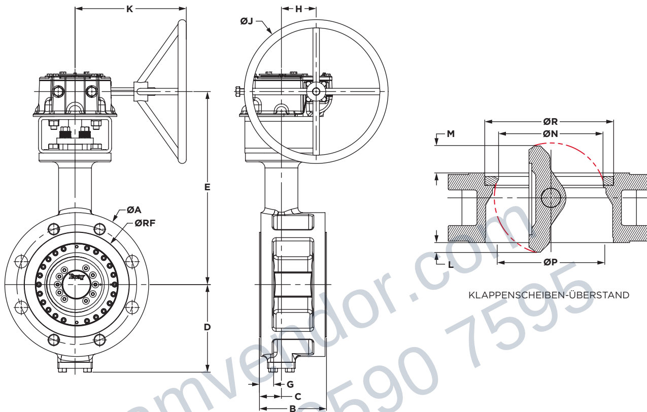
ABMESSUNGEN (mm)
