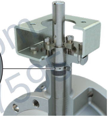
Anillo de sello sólido
