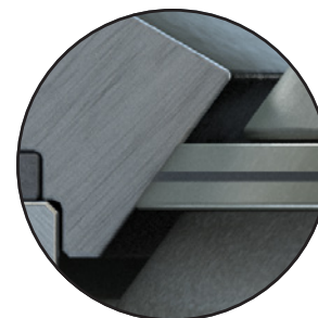
Completamente asentado Una vez asentado, el anillo de sellado se comprime radialmente en el asiento mediante la carga de torque.
