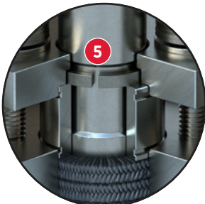
Anillo de prevención de expulsiones Ubicado fuera del límite de presión.
