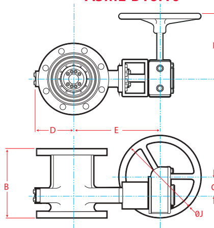
Compuerta API 609 Tabla 3B ASME B16.10
