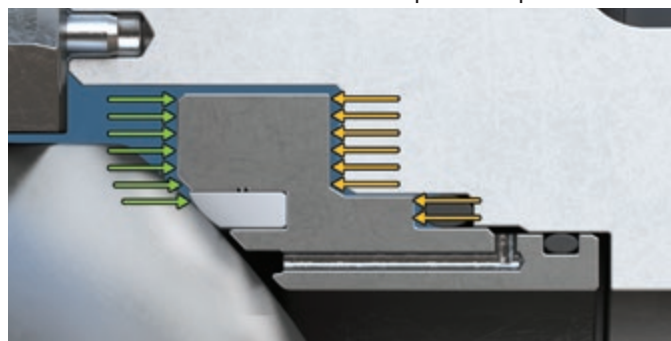
Pressão na cavidade interna no pistão duplo efeito
