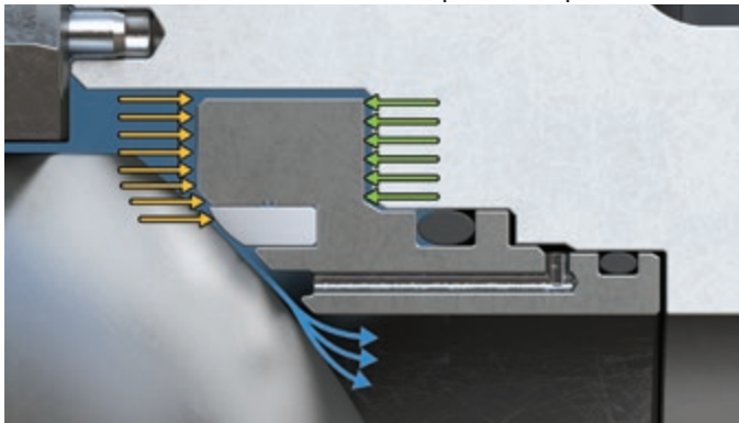
Pressão na cavidade interna no pistão simples efeito
