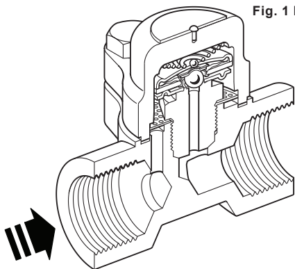
Fig. 1 BPS32
