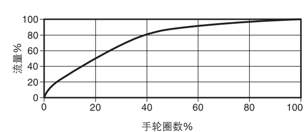
平阀芯BSA2和BSA3
