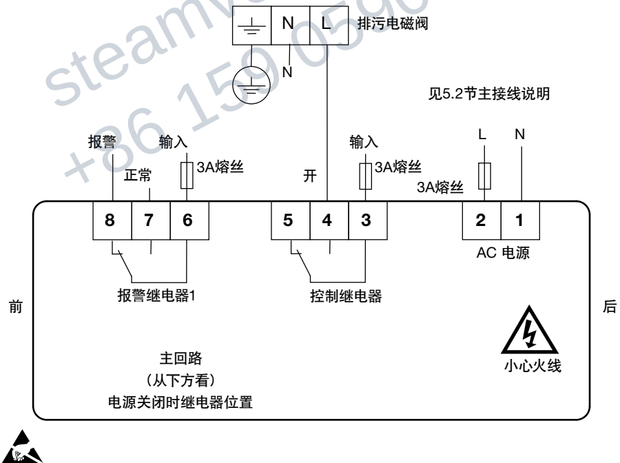
图5 主回路
