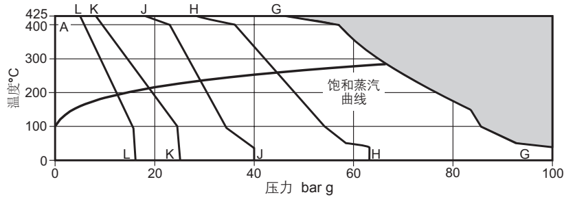
压力/温度范围 - 法兰 DIN
