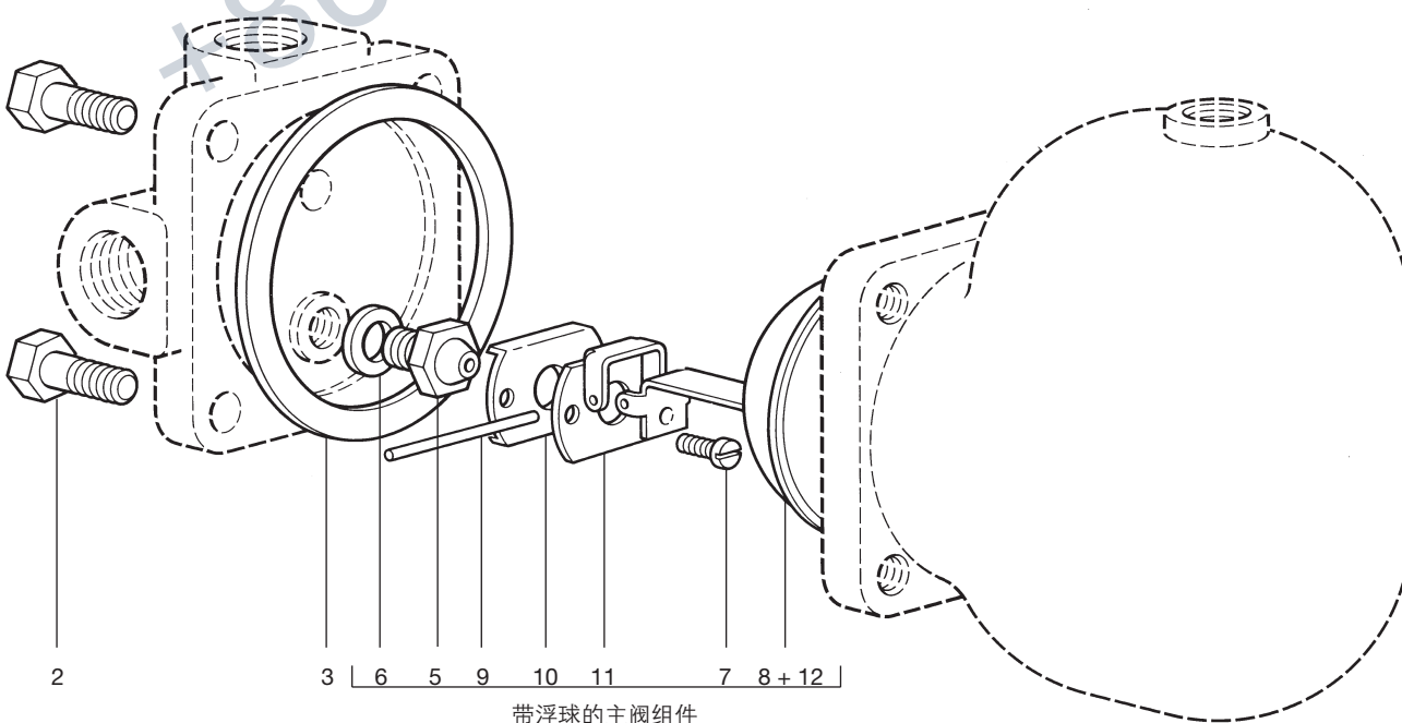
带浮球的主阀组件
