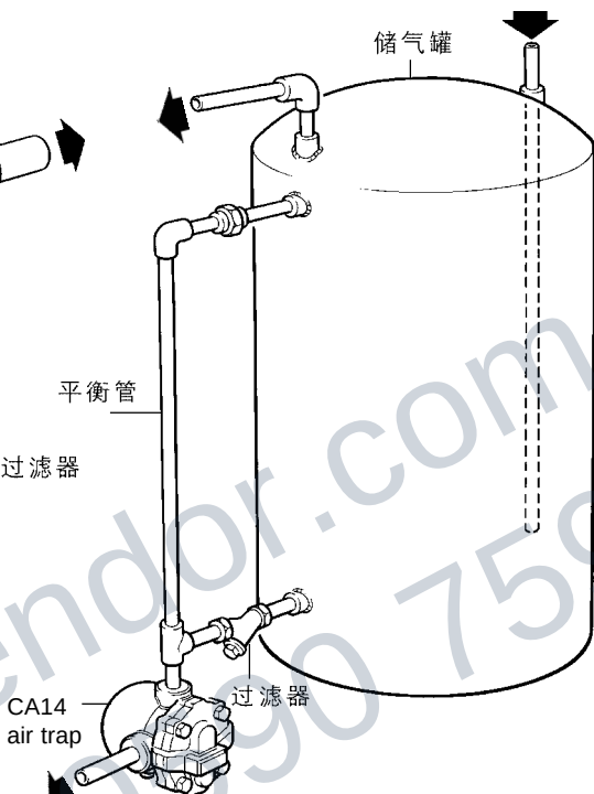
图7：小型储气罐上的疏水阀
