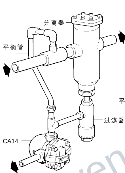
图6：压缩空气主管的汽水分离器上应用的疏水阀
