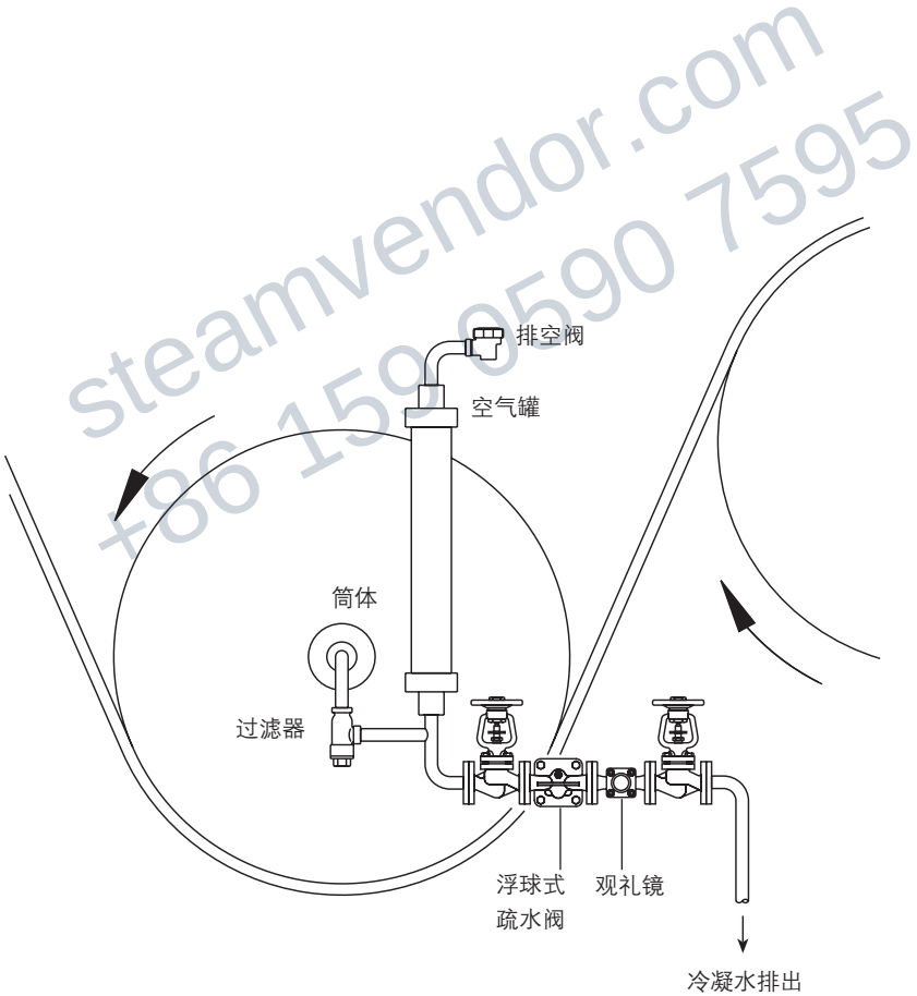
图 6 慢速滚筒疏水系统装置
