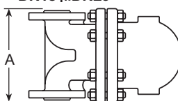
FT47V DN15和DN20
