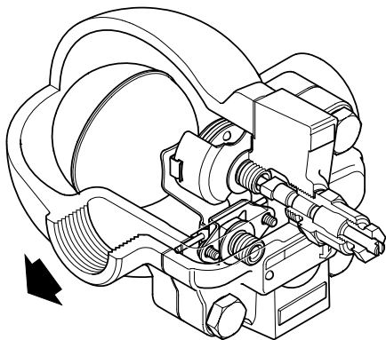
图2 FTGS14-C (R-L)
