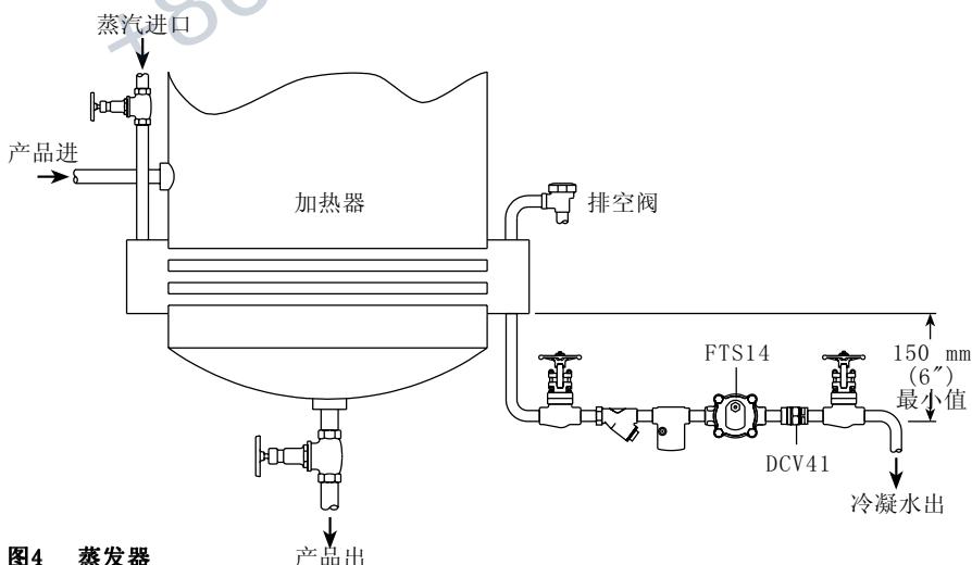
图4 蒸发器
