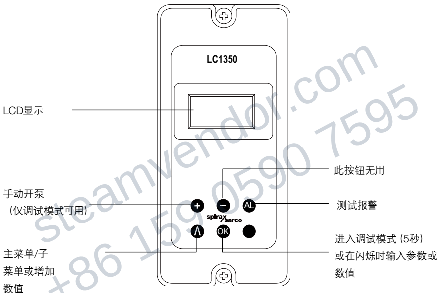
图12 面板显示和键盘
