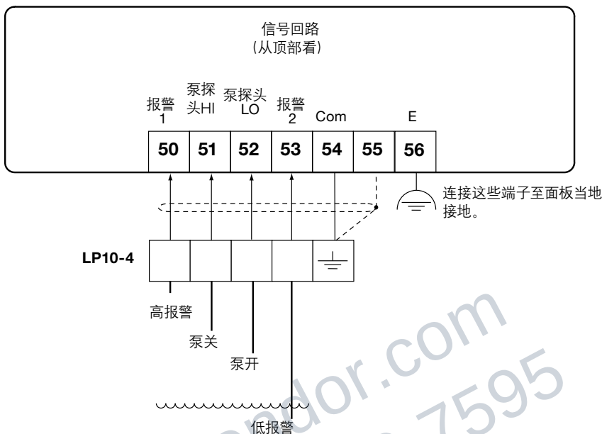
图8 信号回路LP10-4 泵进带一个高报警和一个低报警
