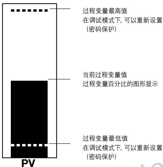
图3 PV(电导率)条形图定义
