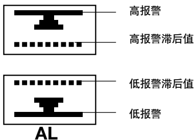
图5 报警条形图定义
