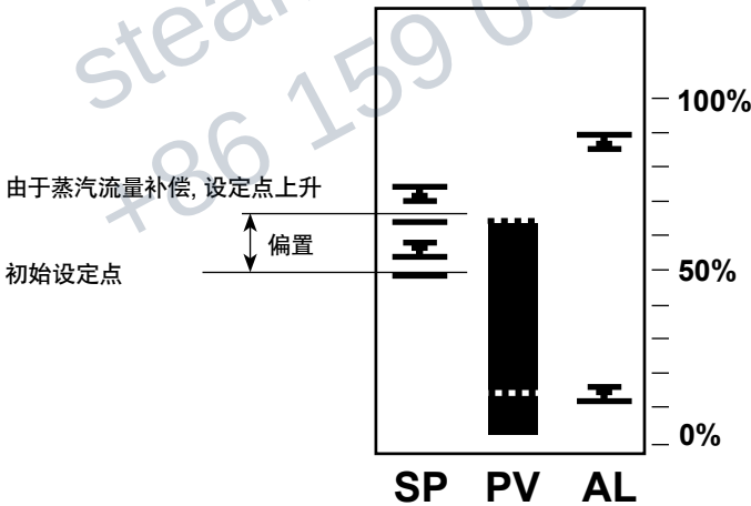
图7 图形显示-有蒸汽流量补偿
