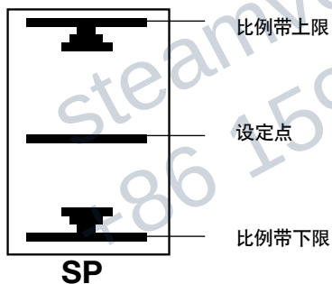
图4 设定点条形图定义
