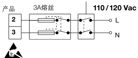
图4 110/120Vac 供电
