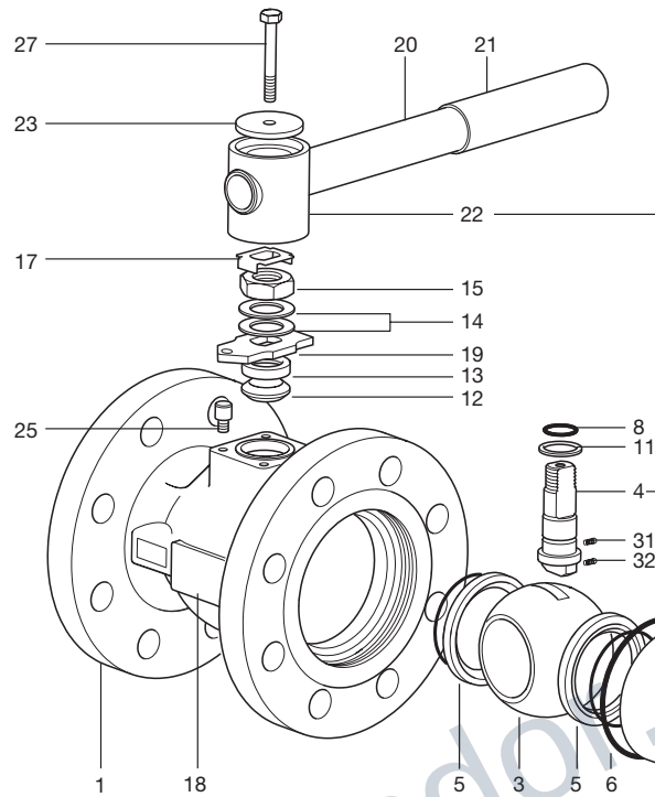
DN65 - DN150
