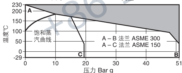
M40Vi2 ISO和M40Vi3 ISO – PTFE阀座
