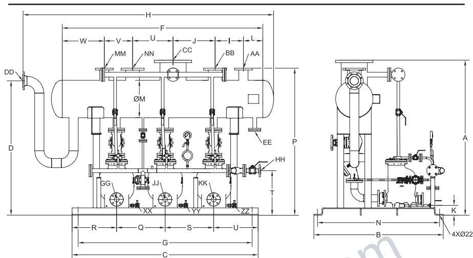
MFP14 DN80三泵组
