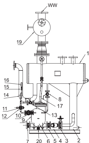
MFP14 DN50, DN80双泵组带选配闪蒸汽回收器
