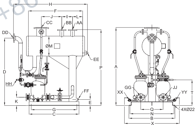
MFP14 DN50, DN80双泵组
