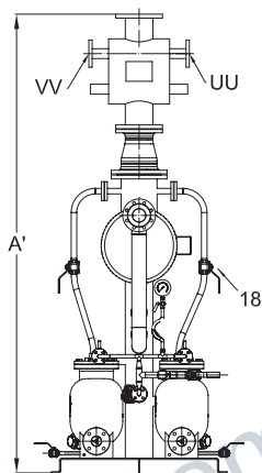
MFP14 DN50, DN80双泵组带选配闪蒸汽回收器
