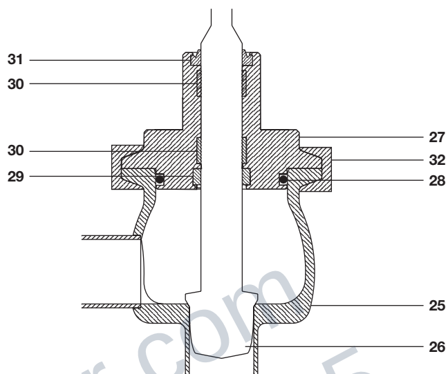
SA 2-通控制阀
